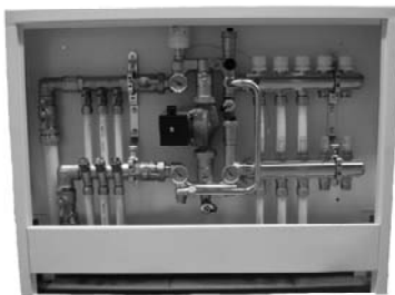
Распределительная система на базе узла COMBI MIX
